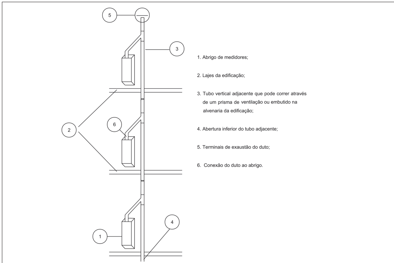
Figura 1: Ventilação de abrigos
