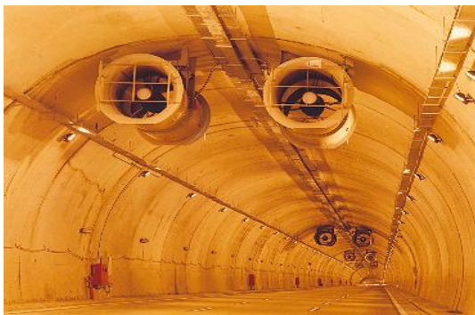
Figura 1 - Sistema de ventilação longitudinal
